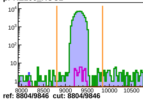
hPRE40_ROC2
