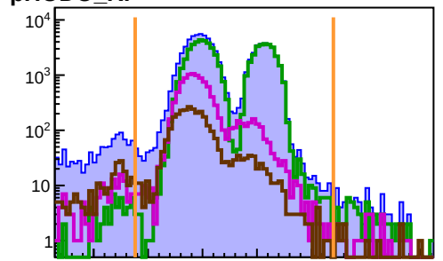
pHODO_RF
