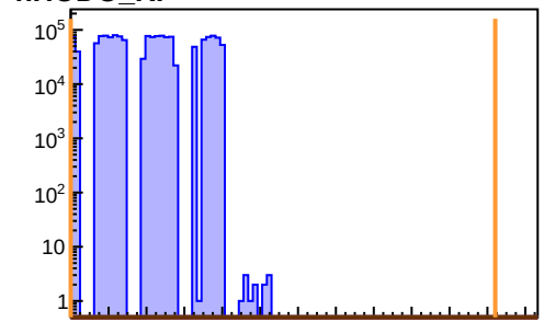
hHODO_RF
