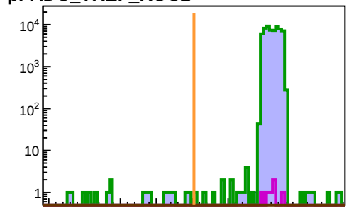
pFADC_TREF_ROC2
