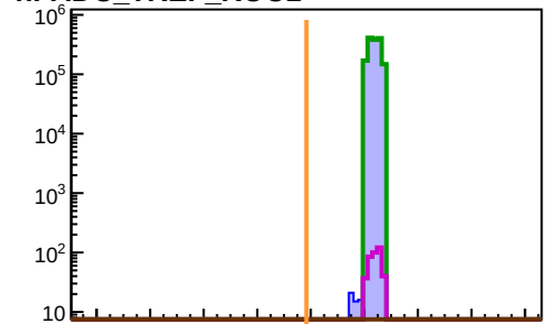
hFADC_TREF_ROC1
