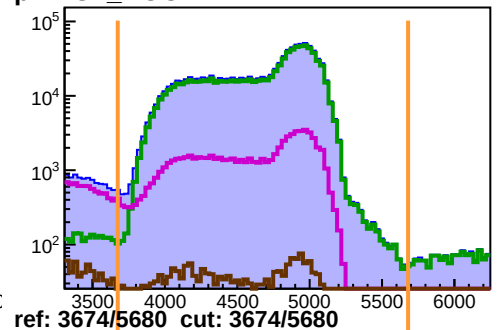
pTRIG5_ROC1
