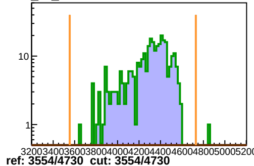
pPRE40_ROC1
