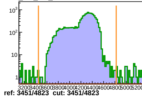
hEL_REAL_ROC1
