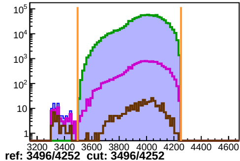
hDCREF3
