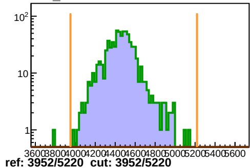
hTRIG2_ROC1
