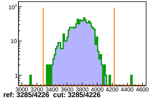
hCER
