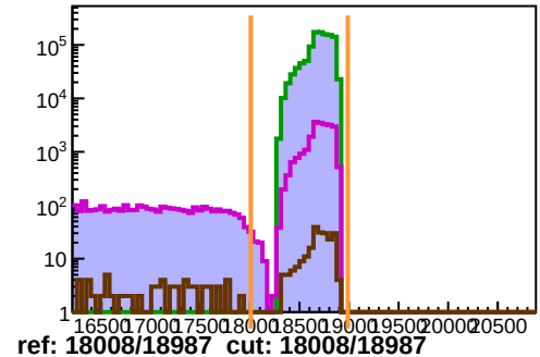
hTRIG3_ROC1
