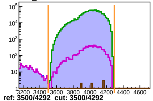
hTRIG1_ROC1
