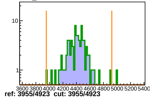
hTRIG3_ROC1
