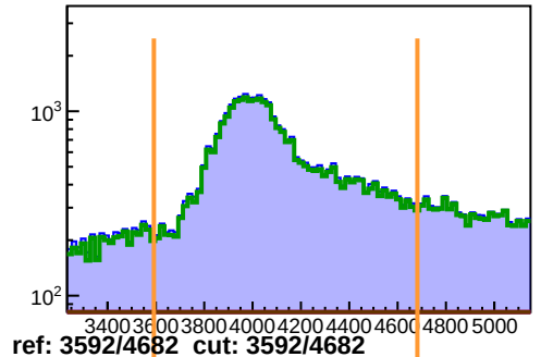
hDCREF2
