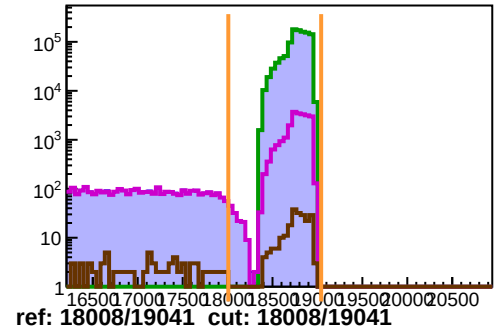
hDCREF4
