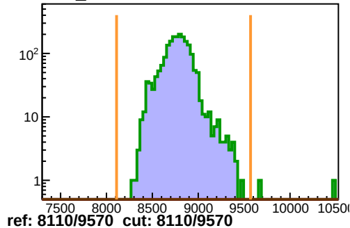
hPRE40_ROC2
