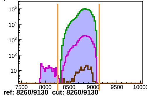
hTRIG1_ROC2
