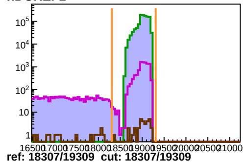
hDCREF4
