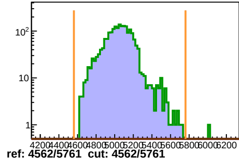
hPRE200_ROC1
