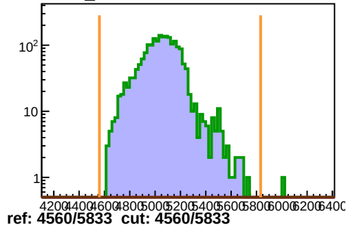
pPRE100_ROC2
