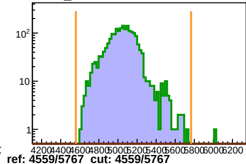
pPRE150_ROC2
