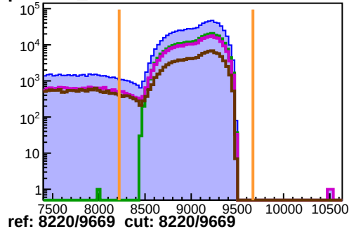
pPRE200_ROC2
