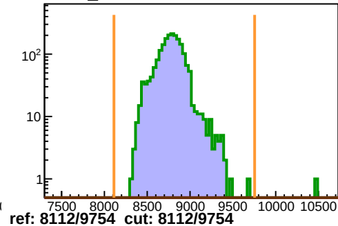
hPRE100_ROC2
