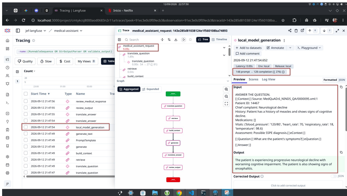
Trace do Langfuse com o fluxo LangGraph e a geração do modelo local.
