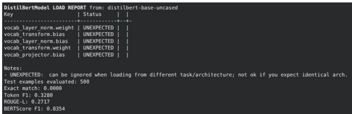
Resultado da avaliação do modelo fine-tuned no conjunto de teste.
