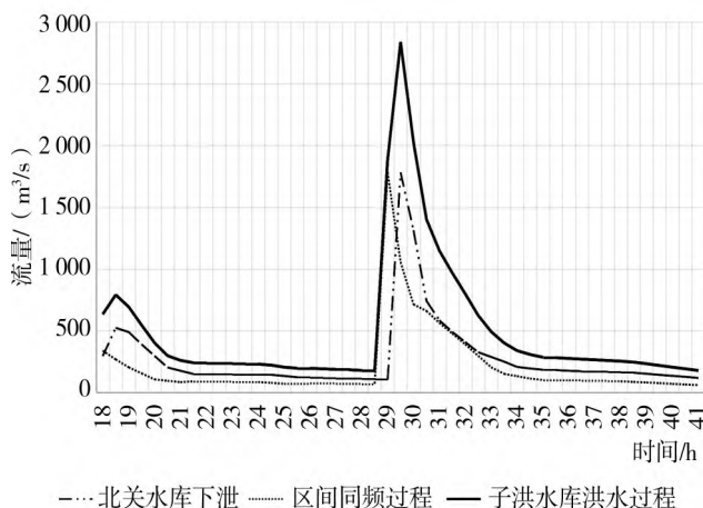
图 1 子洪水库洪水过程线 ( P=0.1\% )
