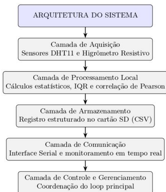
Figura 1: Arquitetura do sistema
