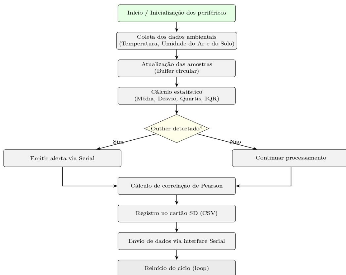
Figura 2: Fluxo de Controle do analisador de solo
