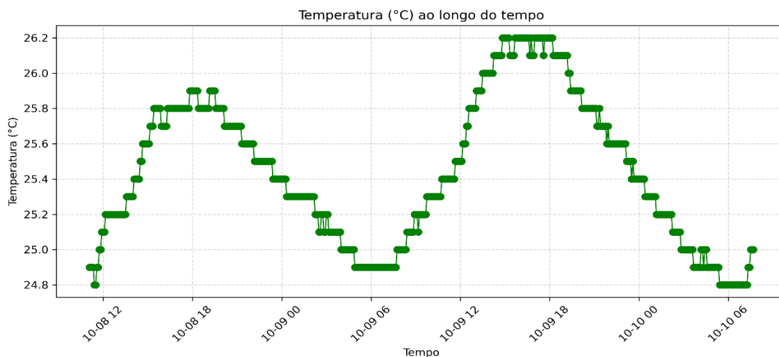
Figura 4: Registro da temperatura obtido no período de coleta.
