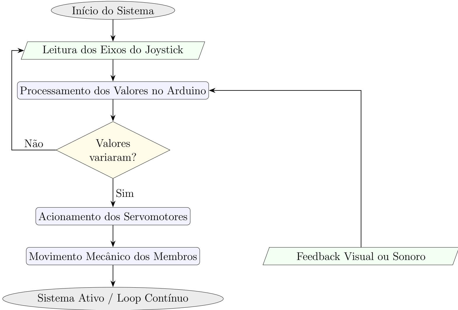
Fluxograma de Controle do Robô Animatrônico
