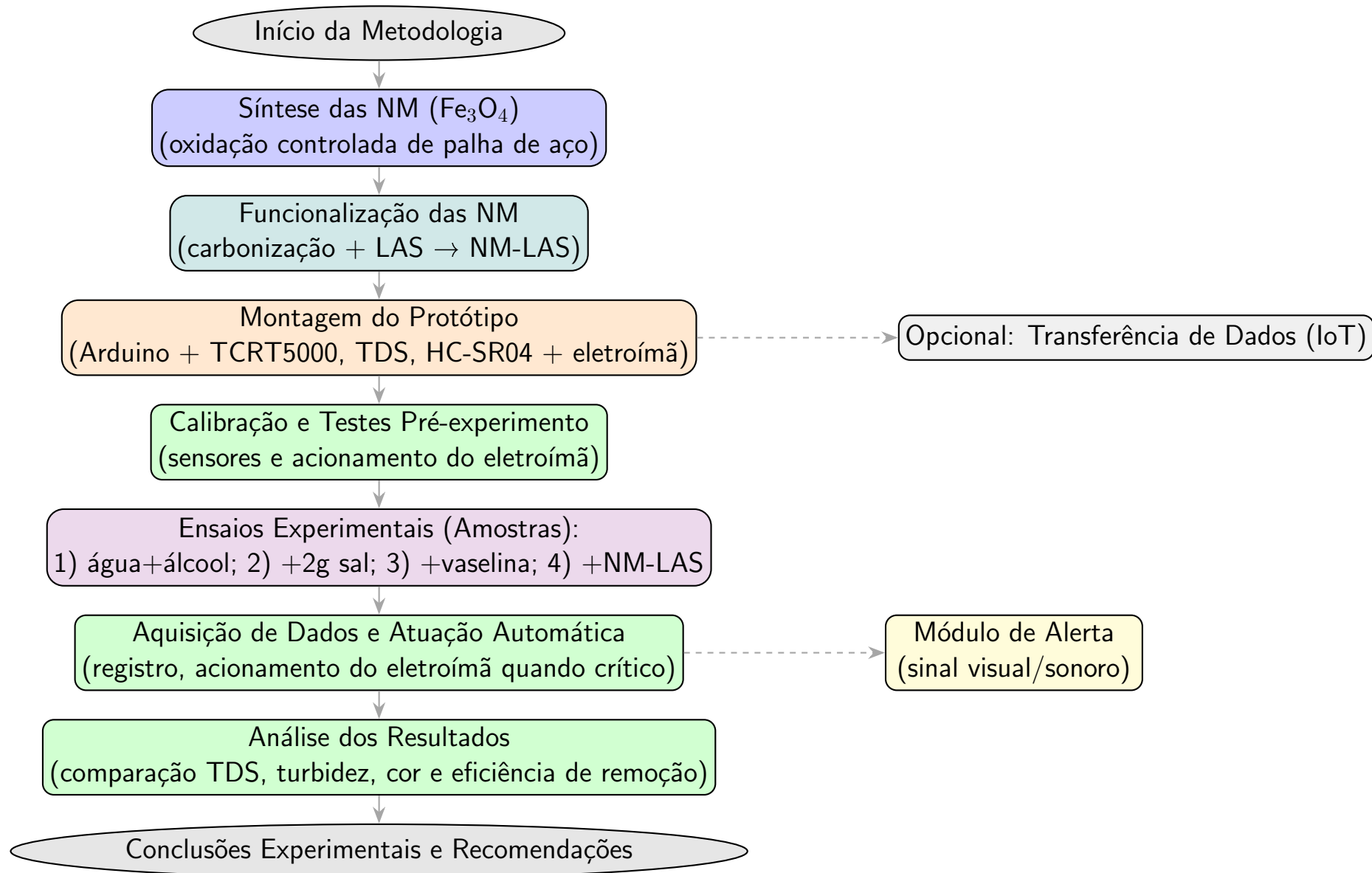
Figura — Fluxograma metodológico: da síntese e funcionalização das nanopartículas até a aquisição automática de dados, ensaios com amostras e análise final.
