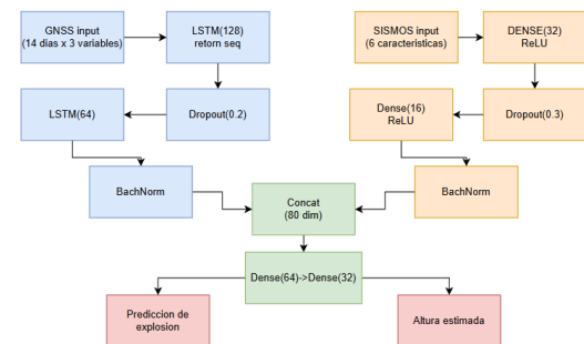
Figure 1: Arquitectura neural multi-modal propuesta. La rama GNSS procesa series temporales de deformación mediante LSTM, mientras que en la rama sísmica procesamos características agregadas. Ambas se combinan para predicción de explosiones e intensidad.
