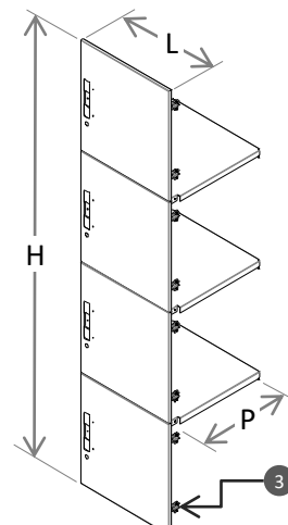
KIT 4 NAVES PARCHE
