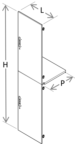
KIT 2 NAVES PARCHE
