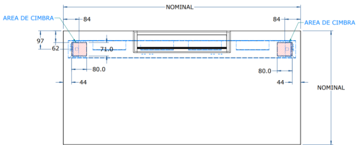
Cimbra desde piso dimensiones en milímetros
