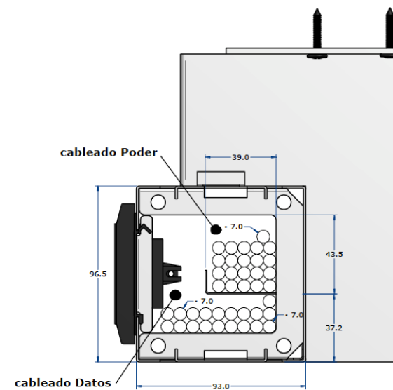
Ducto individual
