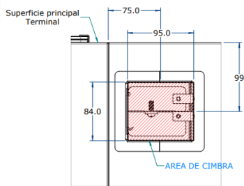
Cimbra desde techo dimensiones en milímetros
