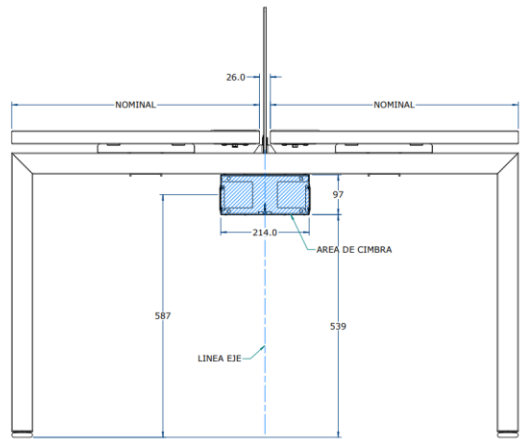
Cimbra desde pared dimensiones en milímetros
