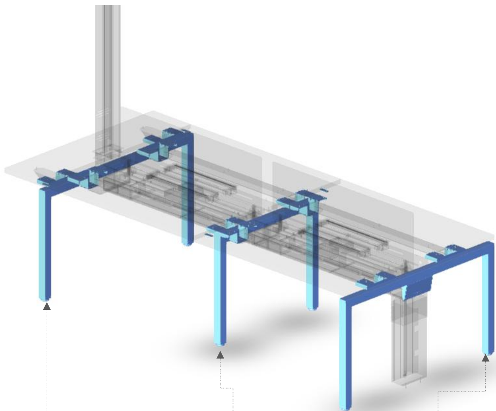
Costado doble intermedio
