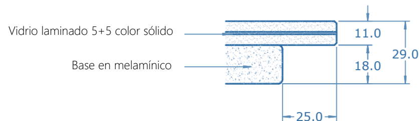
DETALLE SUPERFICIE VIDRIO LAMINADO
