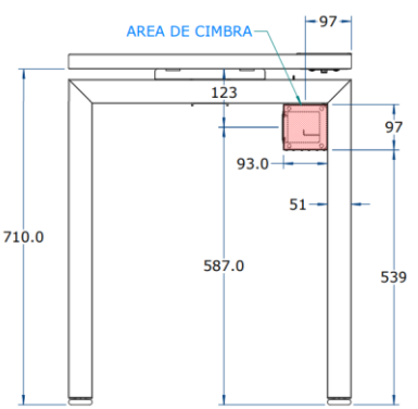
Cimbra desde pared dimensiones en milímetros
