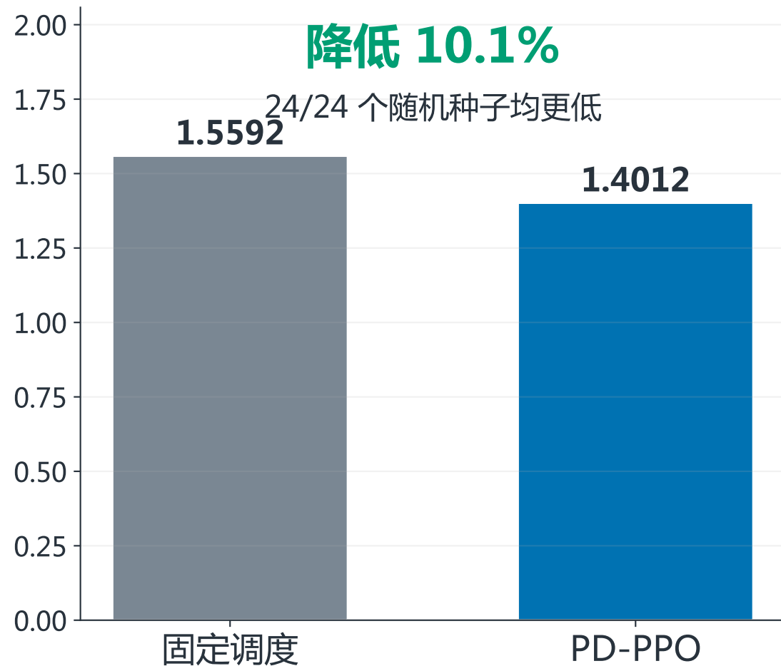
平均多步预测损失
