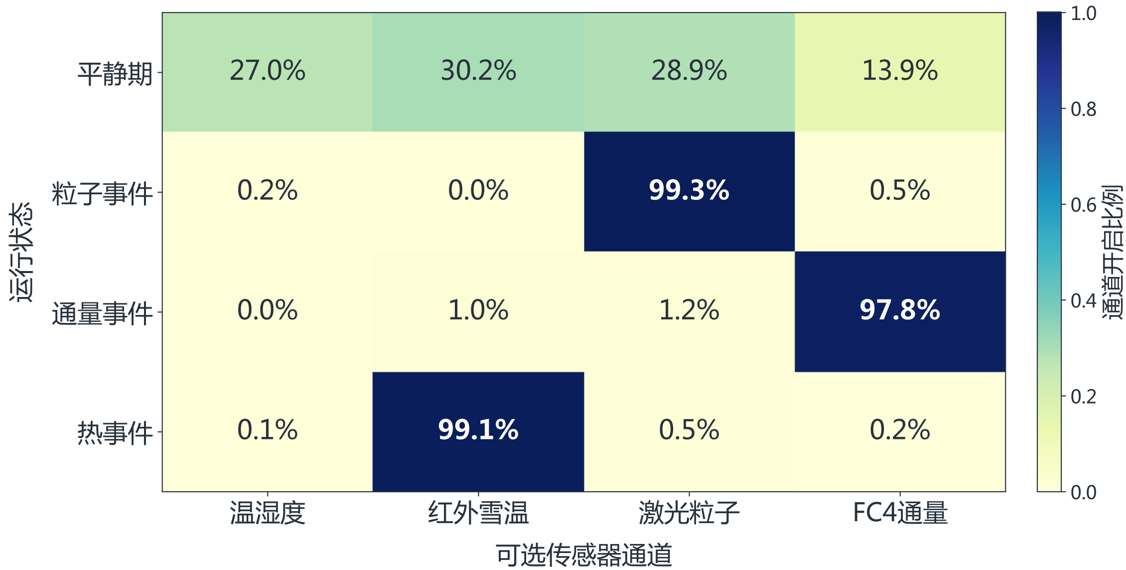
PD-PPO按事件类型分配唯一可选传感器通道
