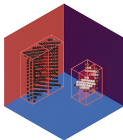
BB Refinement
