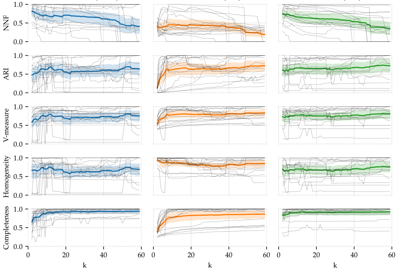
HDBSCAN* (EOM)
