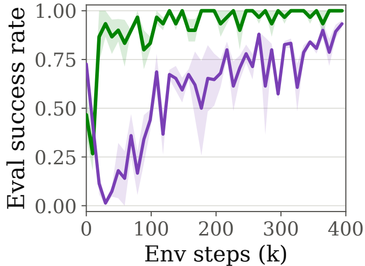
LIBERO-10 · Task 8
