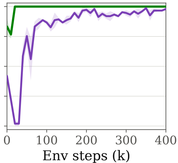
LIBERO-90 · Task 57
