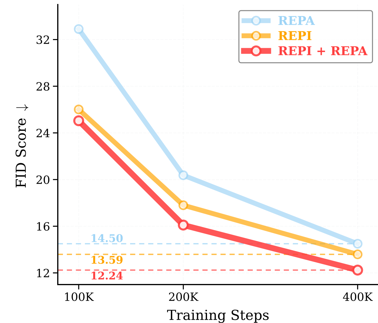
DiT-L/2
