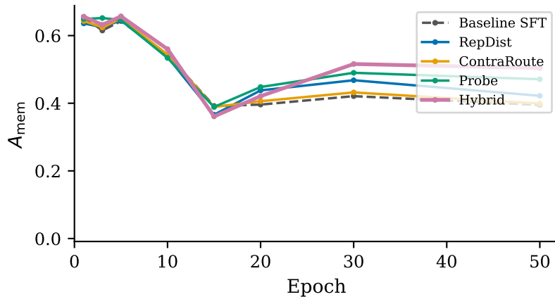
Antares-1B / STaRK-PRIME
