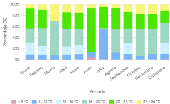
Distribución de rangos de temperatura
