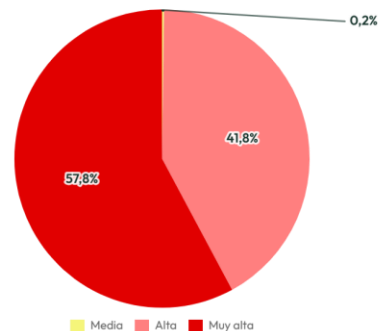
Distribución de las categorías de amenaza por remoción en masa
