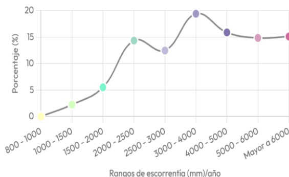
Distribución de la escorrentía por rangos
