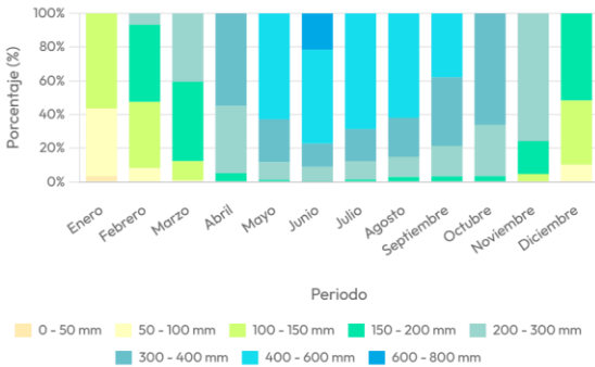
Distribución de rangos de precipitación
