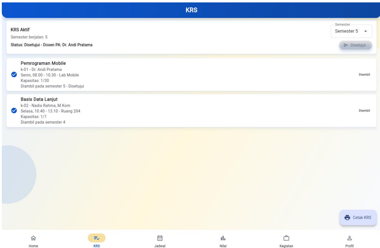
Gambar 3. Halaman KRS mahasiswa dengan status persetujuan, kapasitas kelas, dan tombol cetak KRS.
