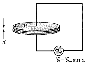
Fig. 32-35 Problem 29.
