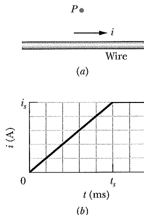
Fig. 32-34 Problem 28.
