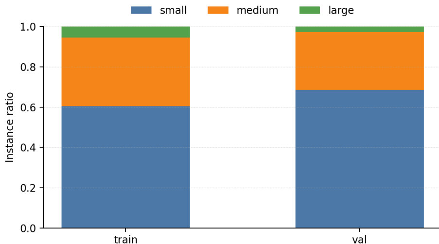
图 3 VisDrone 训练集和验证集目标尺度分布
