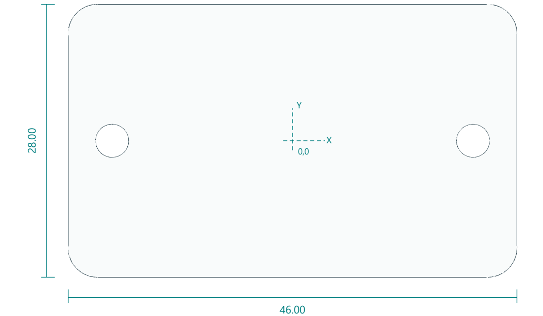
TOP / XY
