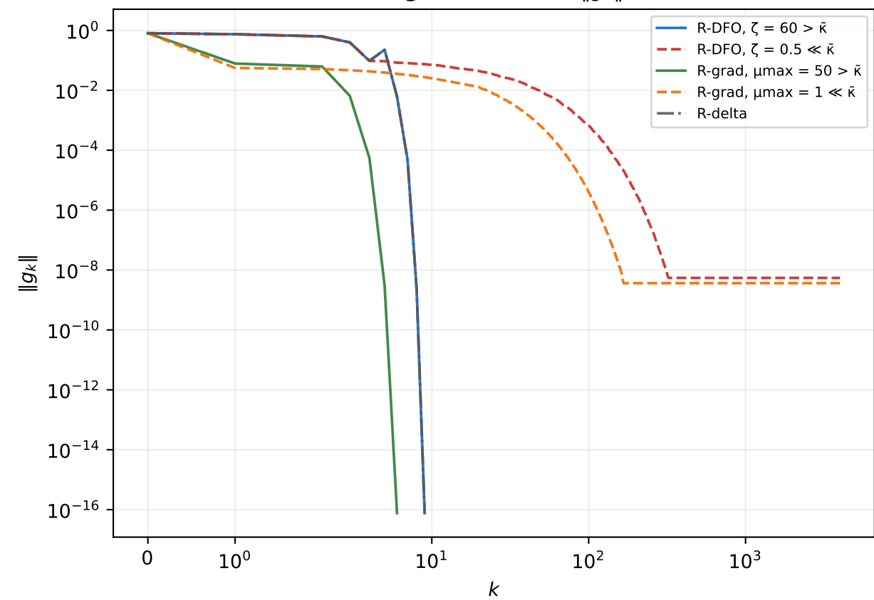
(d) gradient norm \|g_k\|
