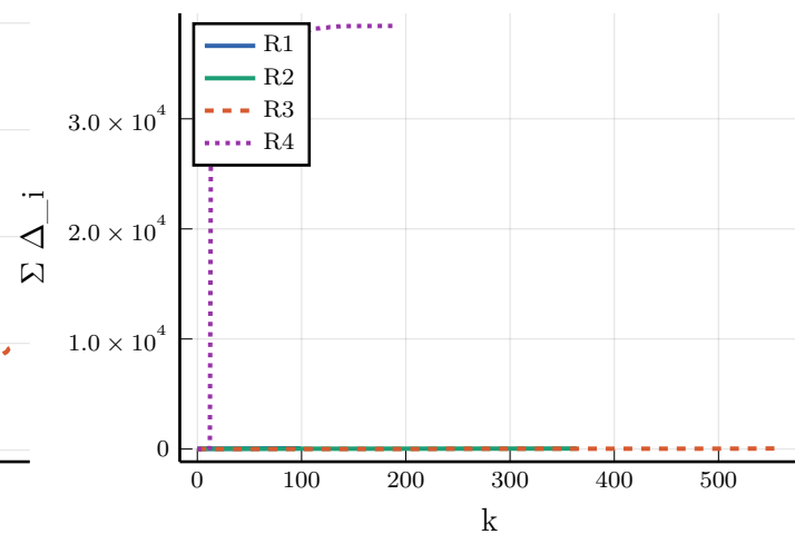
ROSENBRTU
