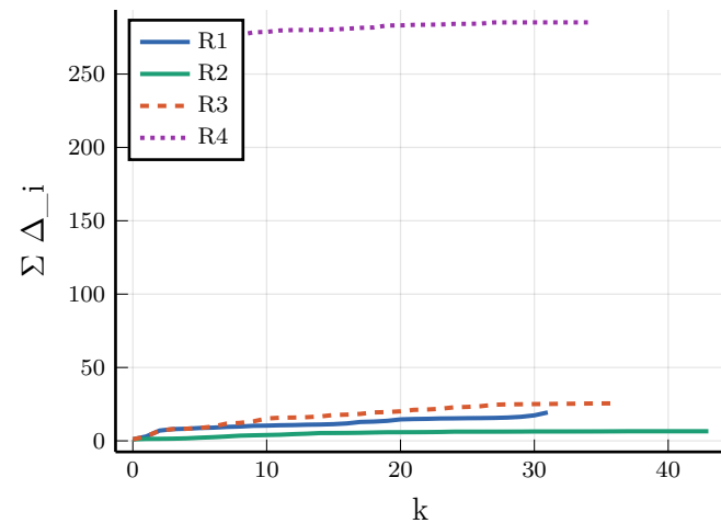
ROSENBRTU
