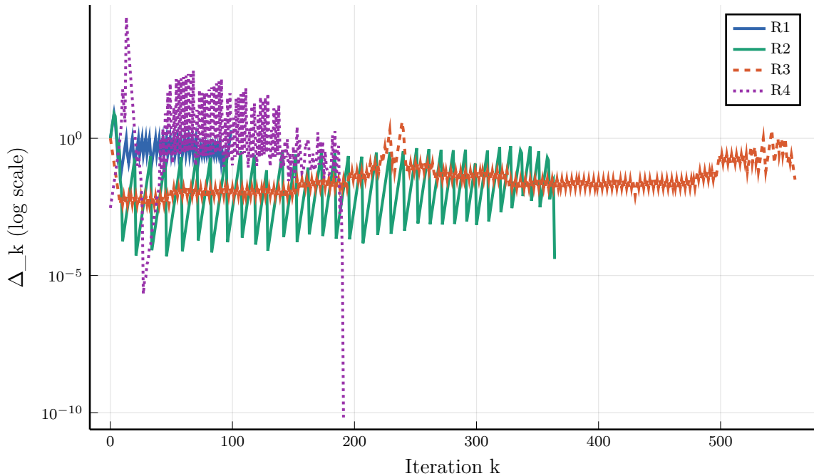
Radius \Delta_k — ROSENBRTU
