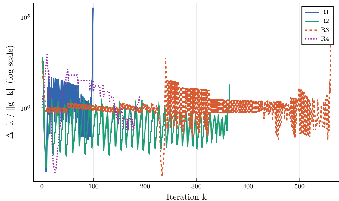
Ratio \Delta\_k / \|g\_k\| — ROSENBRTU
