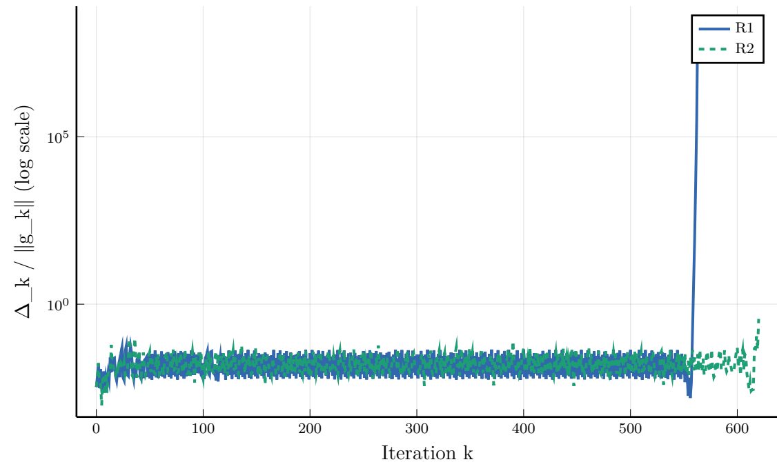
Ratio \Delta\_k / \|g\_k\| — GENROSE
