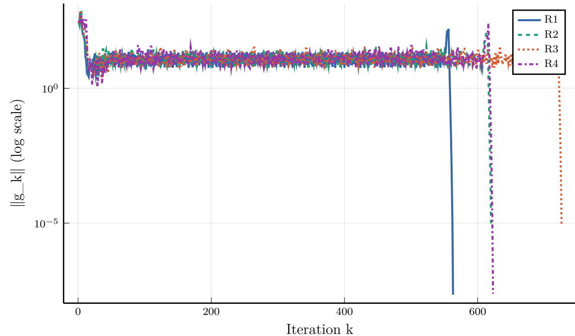
Gradient norm \|g_k\| — GENROSE
