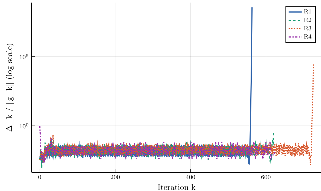
Ratio \Delta\_k / \|g\_k\| — GENROSEB
