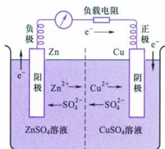
图 8.1 Daniell 电池示意图
