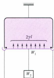
图 13.1 可滑动的金属丝在向上的表面作用力与向下的重力作用下处于平衡
