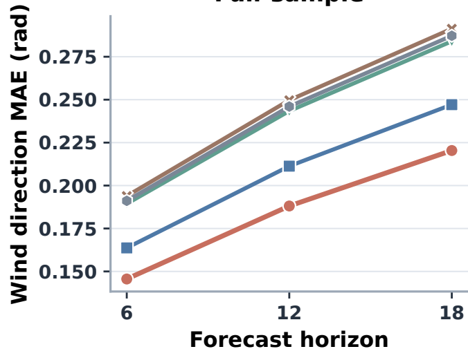
(d) Penmanshiel - Wind direction Full-sample
