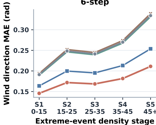
(d) Penmanshiel - Wind direction 6-step
