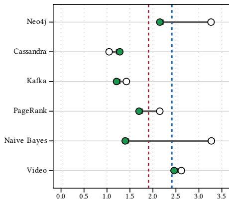
IPC
