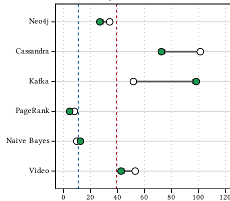
uop-cache (DSB) MPKI
