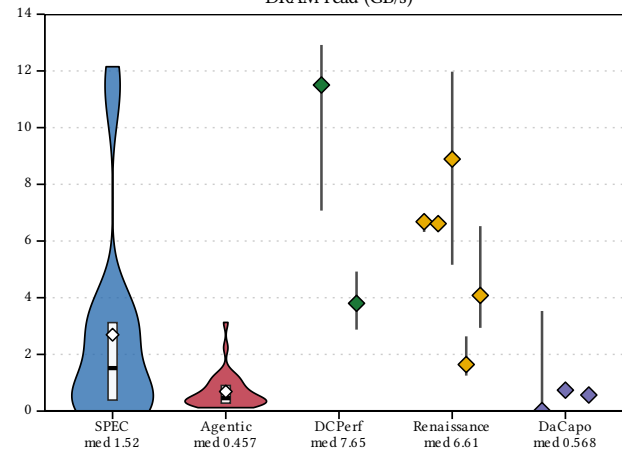
DRAM read (GB/s)
