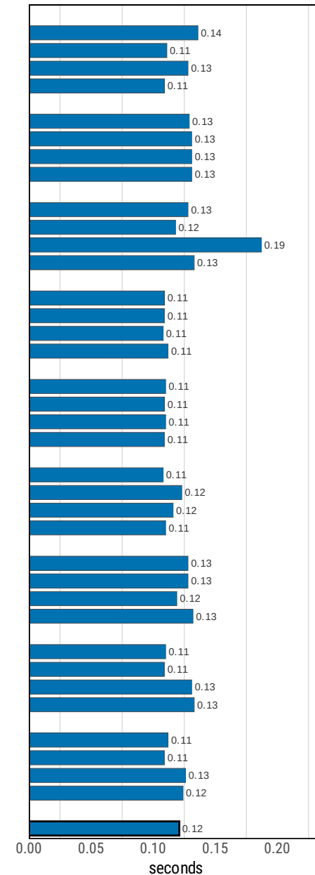
(d) median call duration
