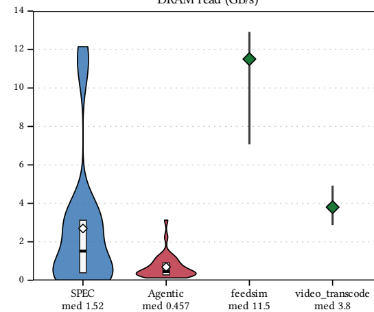
DRAM read (GB/s)
