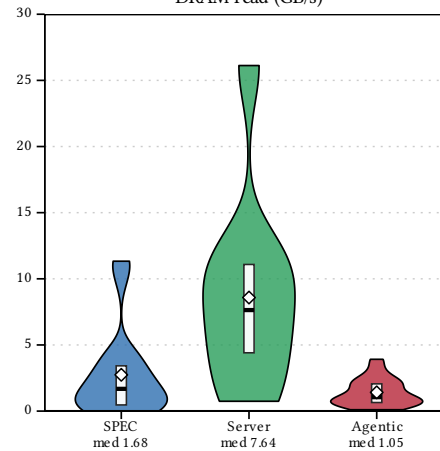
DRAM read (GB/s)
