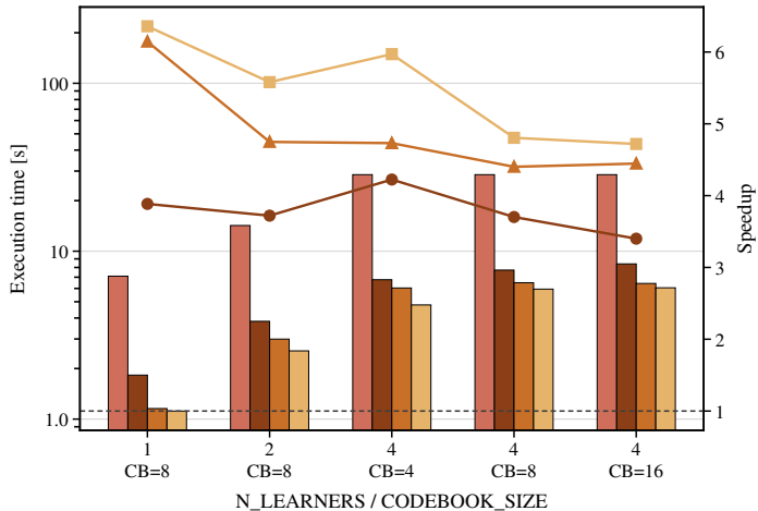
BERT-mini
