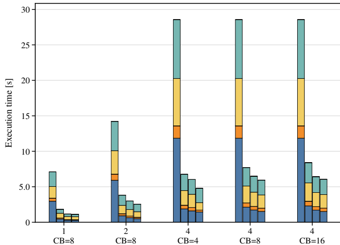
BERT-mini
