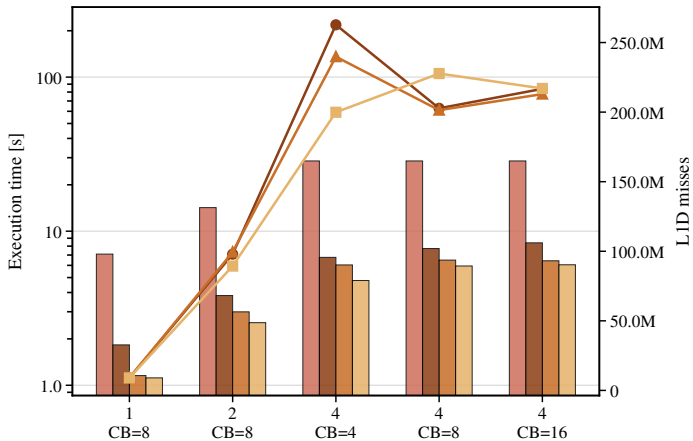
BERT-mini
