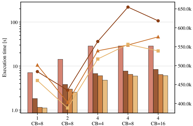
BERT-mini
