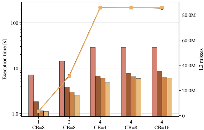
BERT-mini
