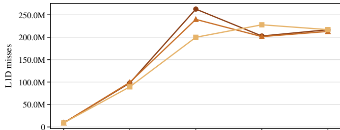
BERT-mini
