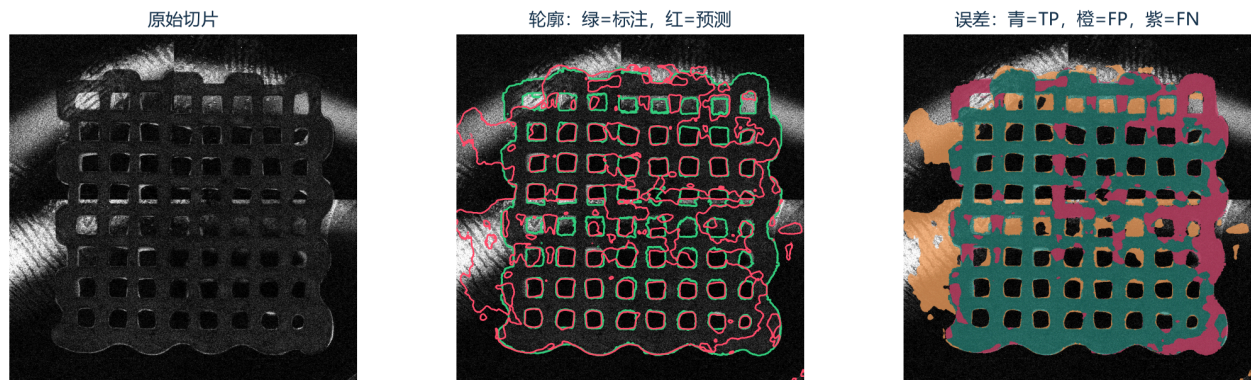
图 5 2_25_XY z=266, slice Dice 0.7573。橙色 FP 和紫色 FN 同时出现，外部高亮结构被误纳入预测。
