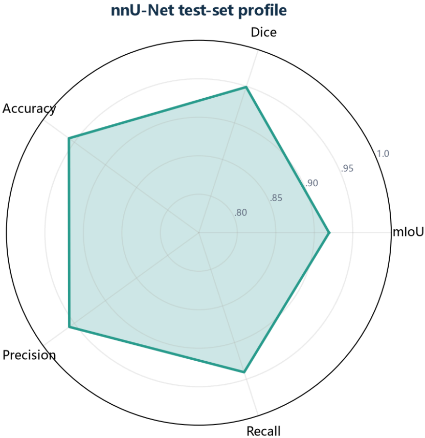
图 2 nnU-Net 最佳 checkpoint 的独立测试指标雷达图。mIoU 为前景/背景两类 IoU 均值，其他指标为 case 宏平均。 雷达图显示五项指标均高于 0.91，Precision 高于 Recall，说明总体更偏向保守预测，漏分风险高于误分风险。这与 2_25_XY 的 FN 可视化相符。另两模型完成后应在同一坐标范围内叠加曲线；如同时考虑速度和参数量，建议另绘 Dice-FPS 散点图，并用点面积表示 Params。
