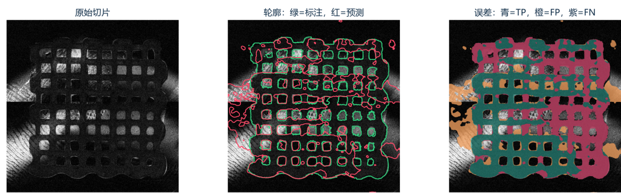
图 4 2_25_XY z=272，slice Dice 0.6285。紫色 FN 较多，表现为目标上部与内部条带漏分。
