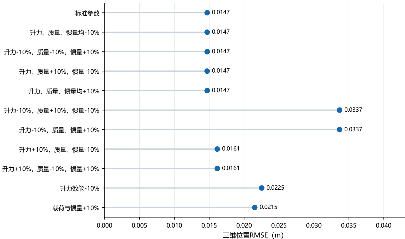
不同参数设置下的跟踪误差
