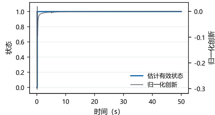
(c) 估计有效状态与创新量
